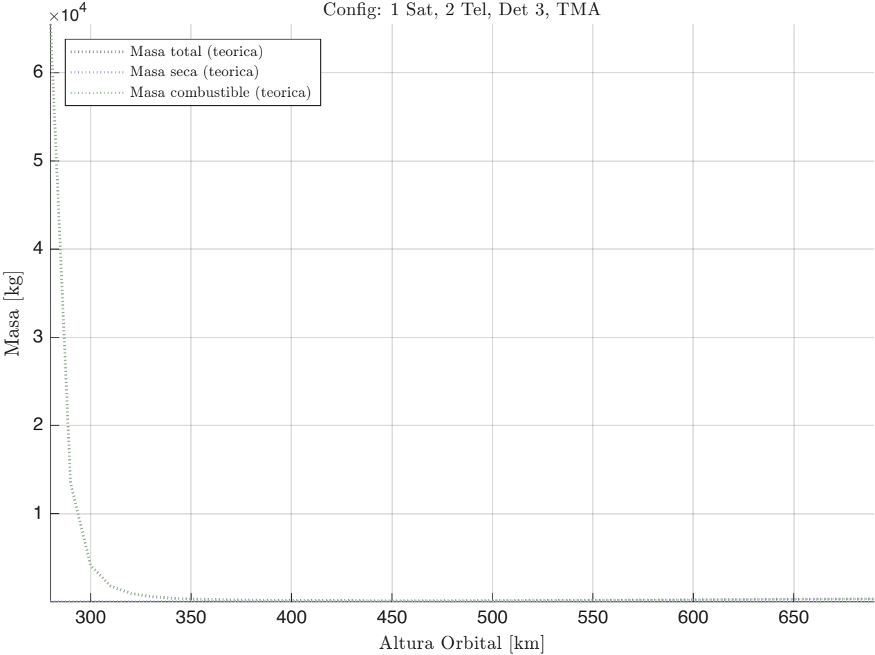
Desglose de Masas vs. Altura Config: 1 Sat, 2 Tel, Det 3, TMA
